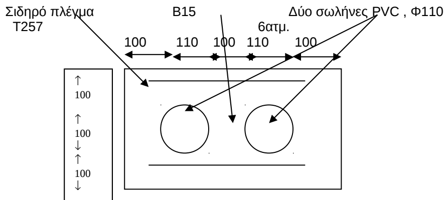
Σχέδιο 2. ΔΙΠΛΟ ΕΡΓΟ ΔΙΑΒΑΣΗΣ
