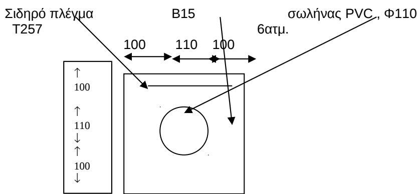
Σχέδιο 1. ΑΠΛΟ ΕΡΓΟ ΔΙΑΒΑΣΗΣ
